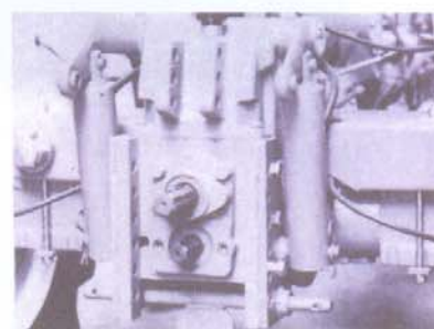
Doble toma de fuerza independiente y sincronizada. Alzamiento con dos cilindros
